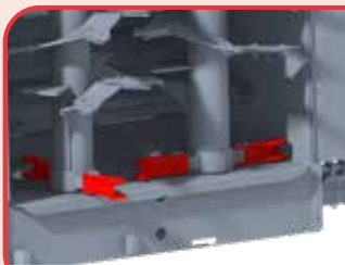
Einklappbare Wurfchaufeln montiert auf Verschleißring für bessere Krümelung.
