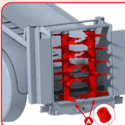
Streuwalzen Ø 900 mm und Windungen von 10 mm Zentralisierte Schmierung der Streuwalzen. Verzinkte Streuklappen mit scharfen Kanten zum Durchtrennen. (A) Verschleißring am Fuß der Streuwalzen.
