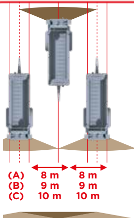
Überlappungszone (variiert je nach Streugut): (A) 8 m (Standard) (B) 9 m mit Weitwurfmessern (C) 10 m mit Streuplatten
